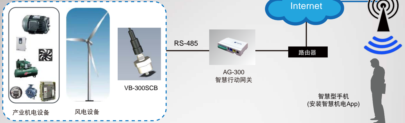
应用架构图
